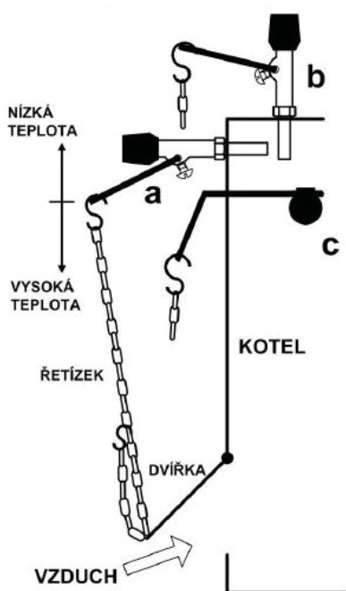
Obr. 2 - montážní polohy regulátoru
