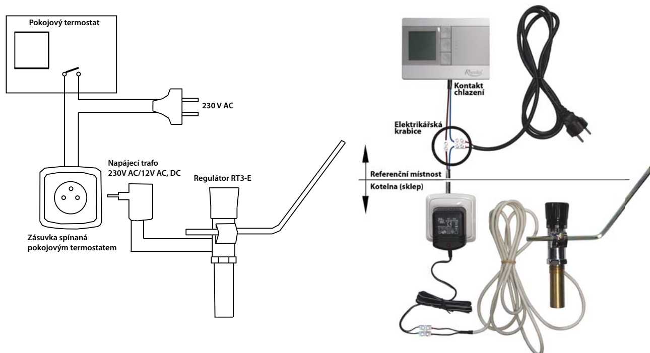
Obr. 5 – termostat spíná 230 V, kontakty musí být dimenzovány na 230 V / 200 mA (zapojení a názorný obrázek)
