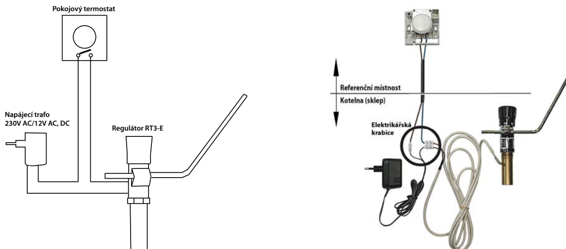
Obr. 4 – termostat spíná 12 V, kontakty musí být dimenzovány na 1 A (zapojení a názorný obrázek)
