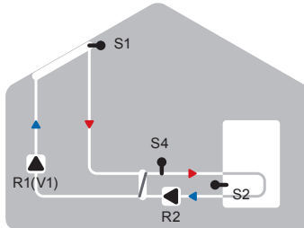
Solární systém s výměníkem
