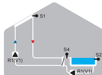
Solární systém s bazénem a výměníkem
