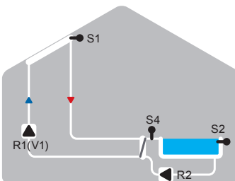
Solární systém s bazénem a výměníkem
