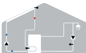
5. Solární systém se zásobníkem s cirkulací
