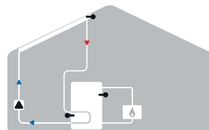
3. Solární systém se zásobníkem a plynový kotel
