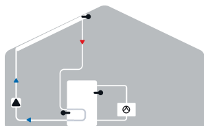
4. Solární systém se zásobníkem a tepelné čerpadlo
