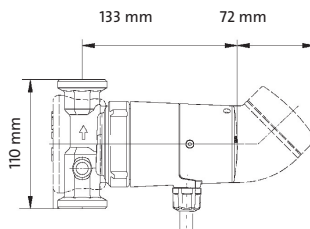
UP 20-14 BX Kompaktní model pro jednoduchou montáž s vnějším závitem G 1 1/4 a celkovou stavební délkou 110 mm
