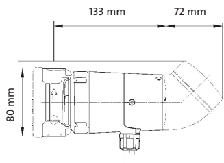
UP 15-14 B Standardní model s vnitřním závitem R 1/2 a celkovou stavební délkou 80 mm
