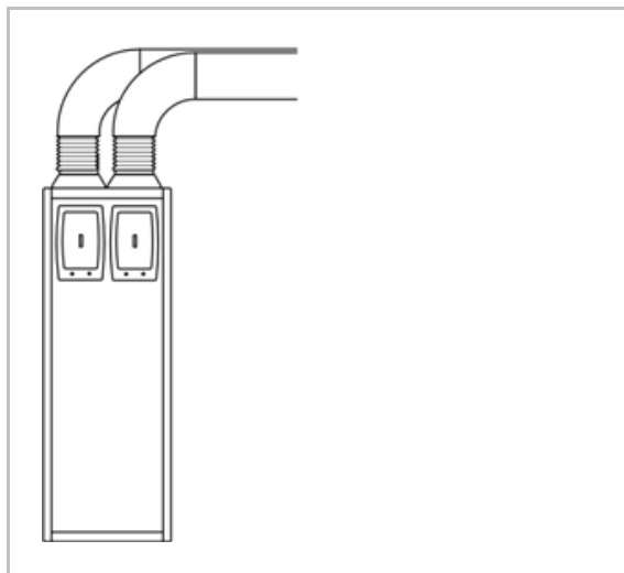
Obr. 22: Připojení potrubí
