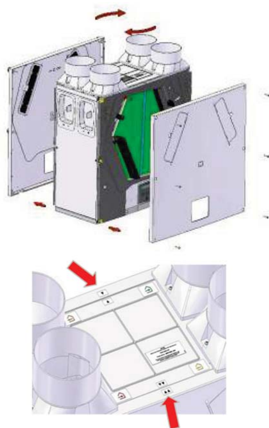
Obr. 3: Instalace přístroje v obrácené poloze
